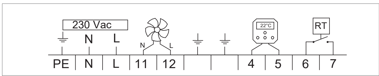
Figuur 26 - Hoofdaansluitingen voor de installatie
