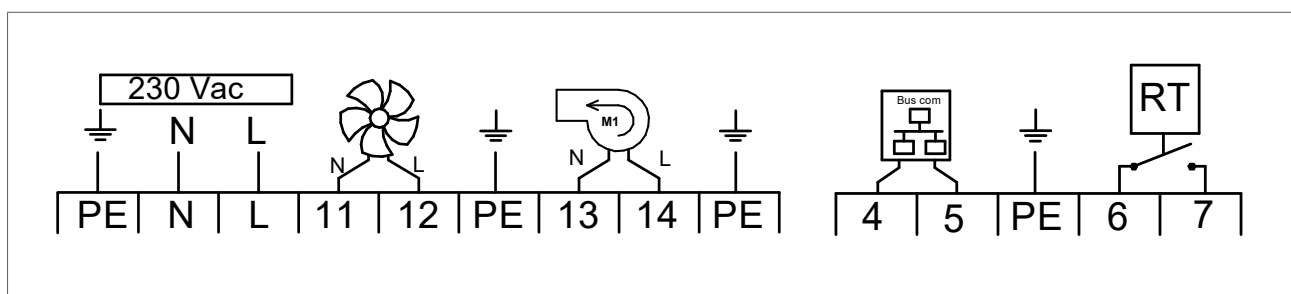
Figuur 14 - Hoofdaansluitingen voor de installatie
