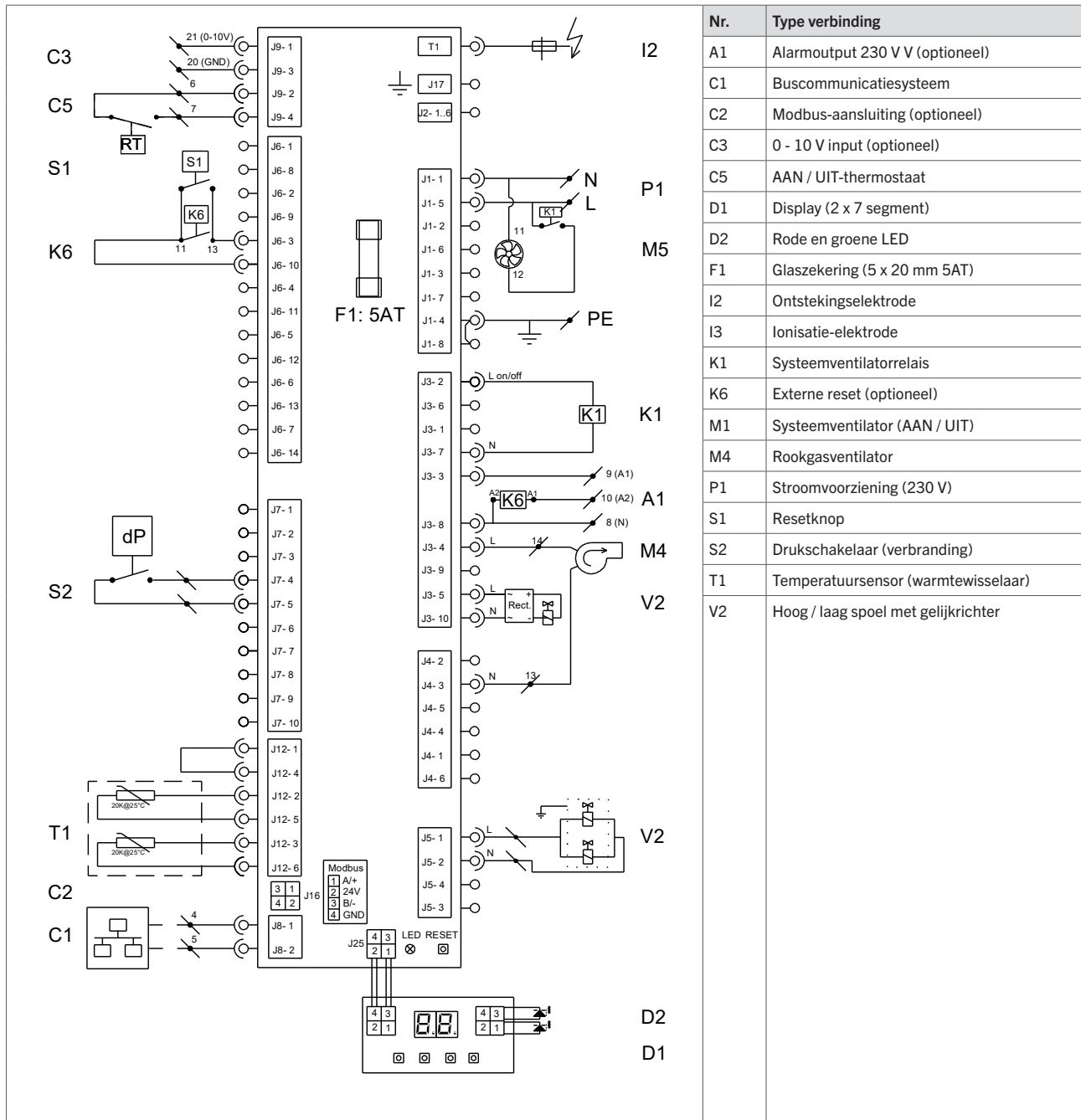
Figuur 13 - Elektrisch schema
