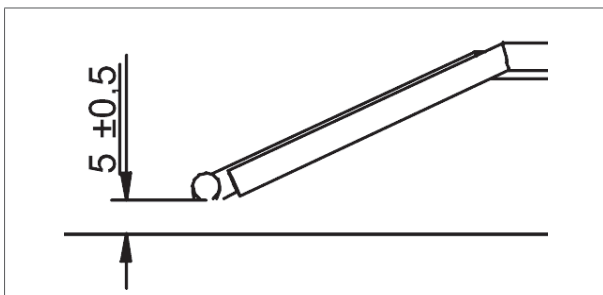
Figuur 23 - Afstand tussen de elektrode en de brander
