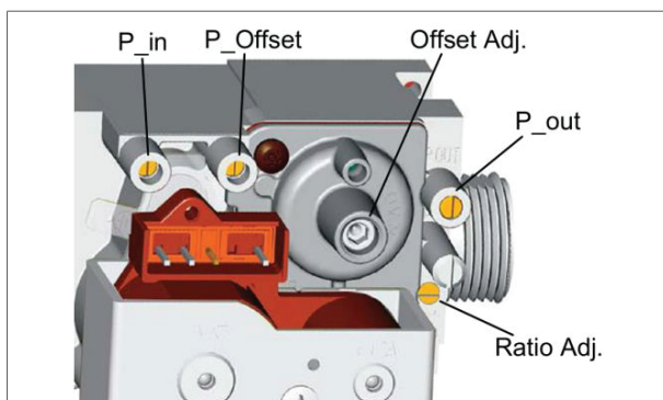
Figuur 22 - Hoofdonderdelen van de gasklep
