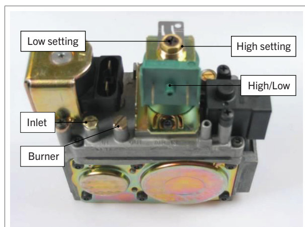
Figuur 12 - Hoofdonderdelen van de gasklep
