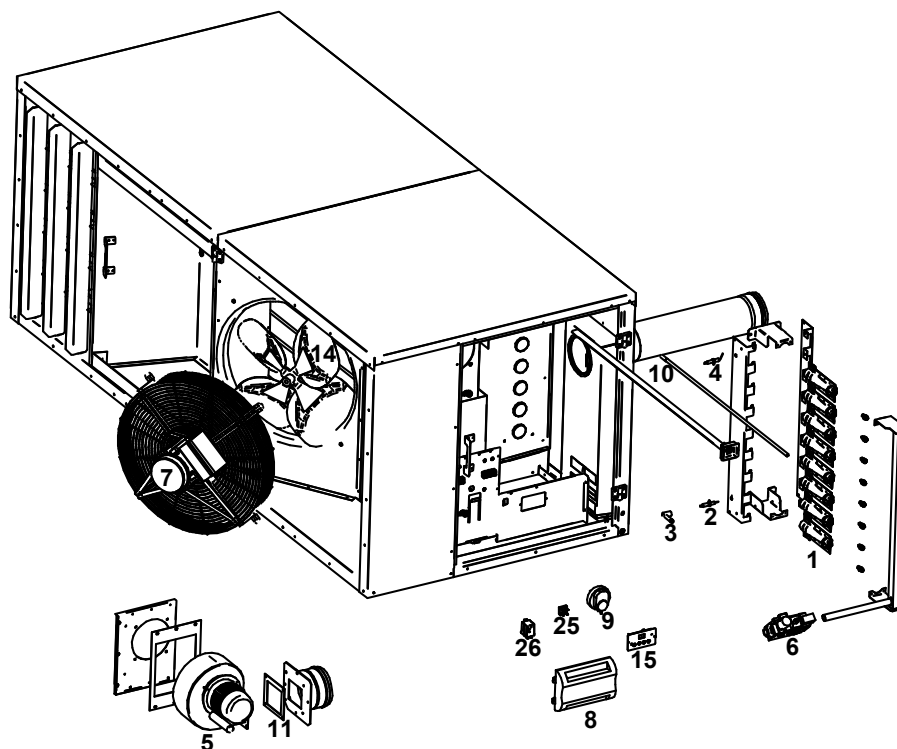
Figuur 16 - Exploded view van de DXE
