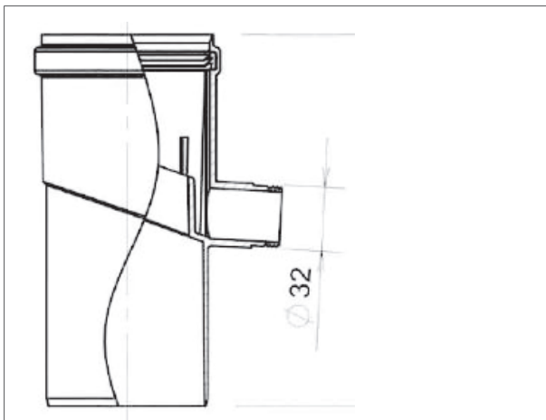
Figuur 14 - Condensaatafvoer
