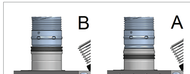
Figuur 16 - Afdichting voor bescherming tegen water
