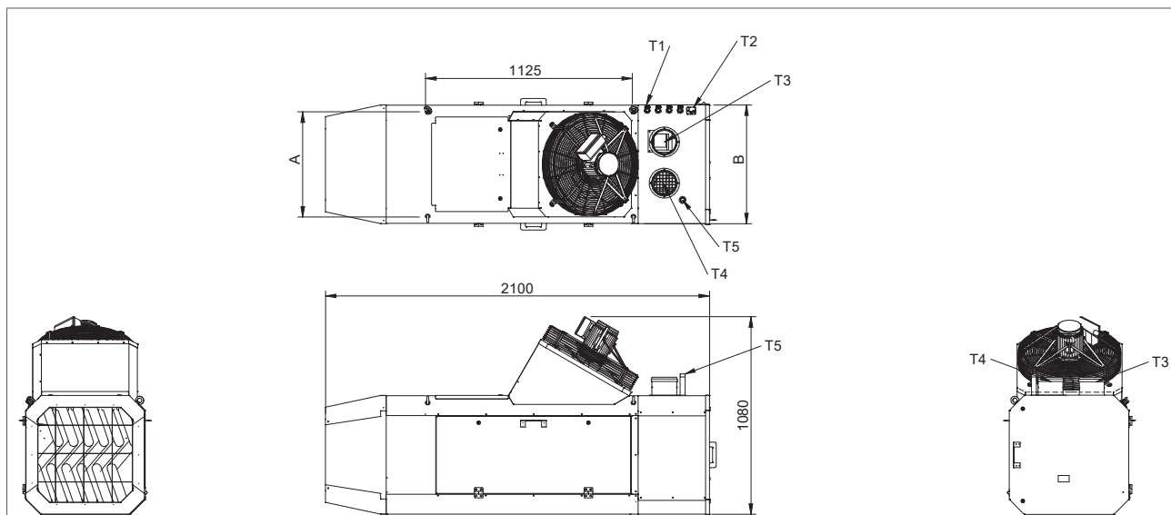
Figuur 1 - Afmetingen van de DXC
