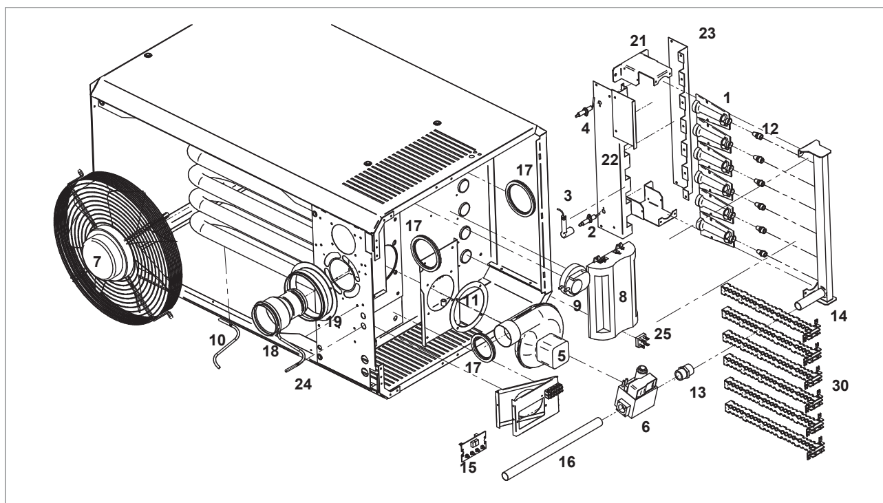
Figuur 29 - Explosietekening van de TR24 - TR50
