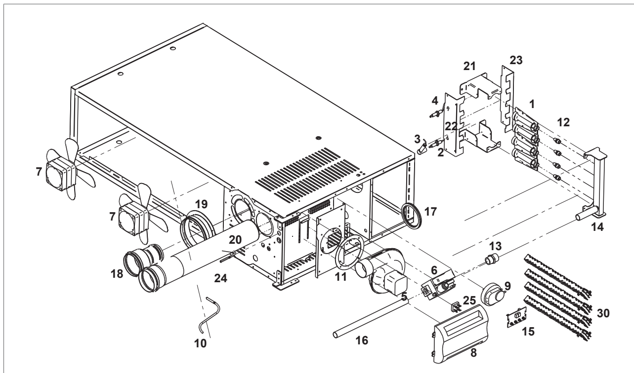
Figuur 28 - Explosietekening van de TR10 - TR20
